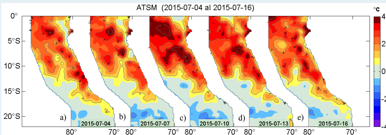
Figura 2. Anomalías de la temperatura superficial del agua (°C) en el mar peruano los días a) 04, b) 07, c) 10, d) 13 y e) 16 de julio. Datos: AVHRR/NOAA. Procesamiento: IMARPE.
