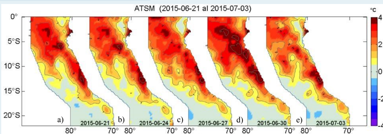
Figura 2. Anomalías de la temperatura superficial del agua (°C) en el mar peruano los días: a) 21, b) 24, c) 27, d) 30 de junio y e) 03 de julio. Datos: AVHRR/NOAA. Procesamiento: IMARPE.
