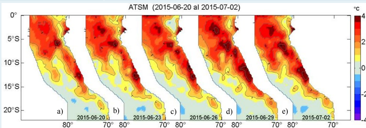
Figura 2. Anomalías de la temperatura superficial del agua (°C) en el mar peruano los días a) 20, b) 23, c) 26, d) 29 de junio y e) 02 de julio. Datos: AVHRR/NOAA. Procesamiento: IMARPE.
