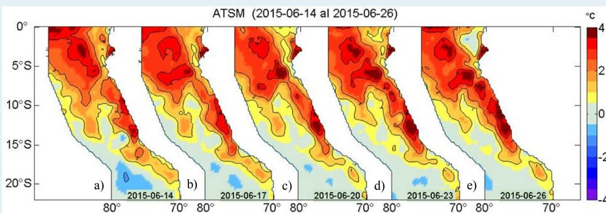
Figura 2. Anomalías de la temperatura superficial del agua ( ^{\circ}\text{C} ) en el mar peruano los días: a) 14, b) 17, c) 20, d) 23 y e) 26 de junio. Datos: AVHRR/NOAA. Procesamiento: IMARPE.
