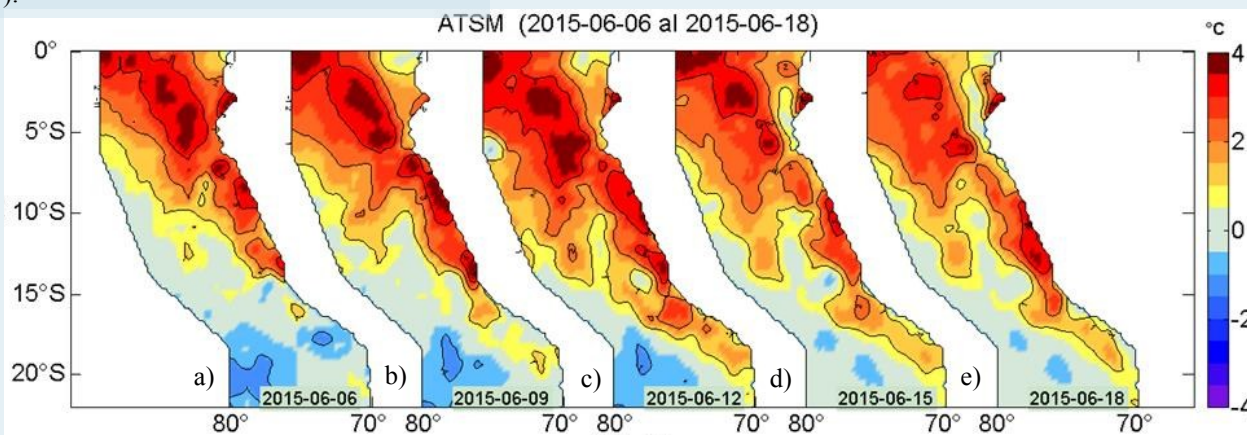
Figura 2. Anomalías de la temperatura superficial del agua (°C) en el mar peruano los días a) 06, b) 09, c) 12, d) 15 y e) 18 de junio. Datos: AVHRR/NOAA. Procesamiento: IMARPE.
