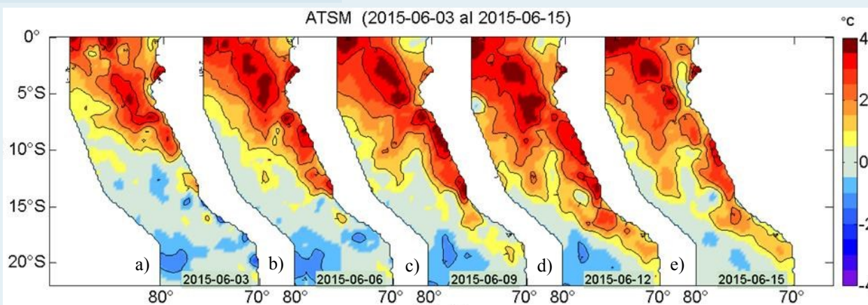
Figura 2. Anomalías de la temperatura superficial del agua (°C) en el mar peruano los días a) 03, b) 06, c) 09, d) 12 y e) 15 de junio. Datos: AVHRR/NOAA. Procesamiento: IMARPE.
