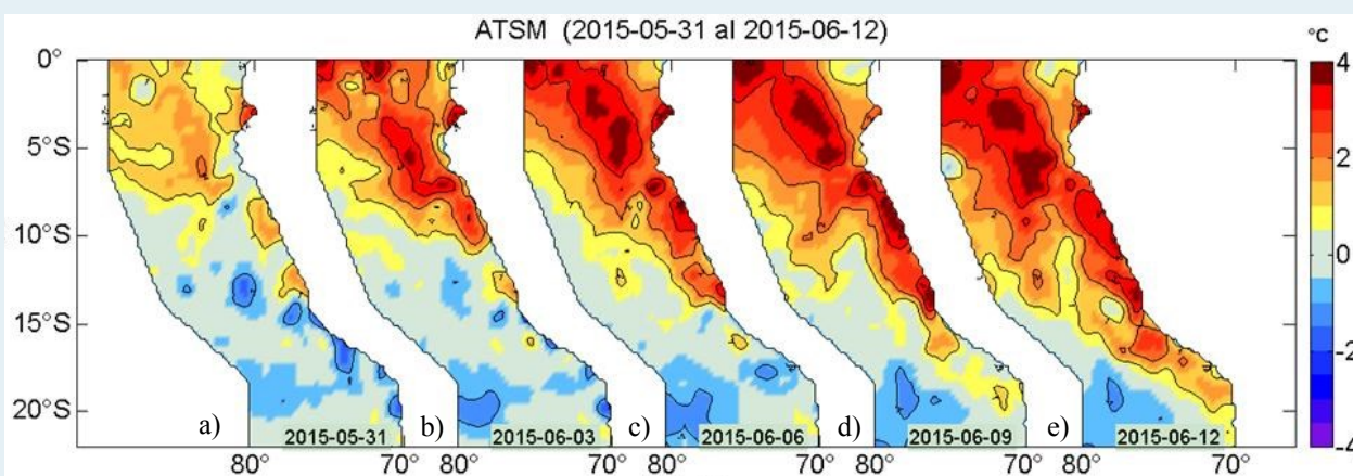
Figura 2. Anomalías de la temperatura superficial del agua (°C) en el mar peruano los días a) 31 de mayo, b) 03, c) 06, d) 09 y e) 12 de junio. Datos: AVHRR/NOAA. Procesamiento: IMARPE.
