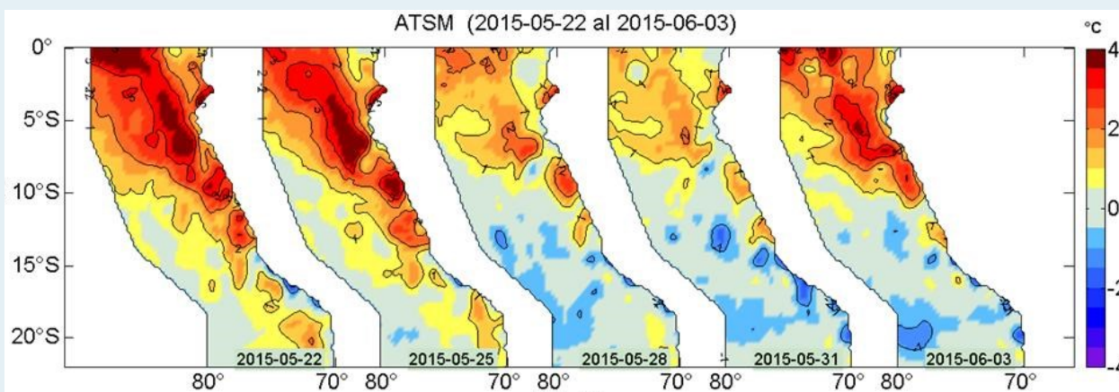
Figura 2. Anomalías de la temperatura superficial del agua (°C) en el mar peruano los días 22, 25, 28, 31 de mayo y 03 de junio. Datos: AVHRR/NOAA. Procesamiento: IMARPE.
