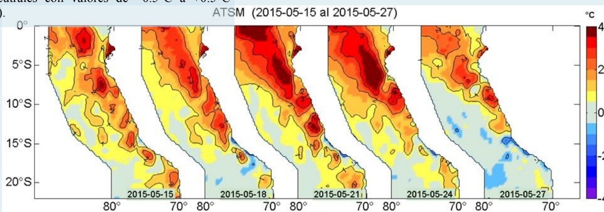
Figura 2. Anomalías de la temperatura superficial del agua (°C) en el mar peruano los días 15, 18, 21, 24 y 27 de mayo. Datos: AVHRR/NOAA. Procesamiento: IMARPE.
