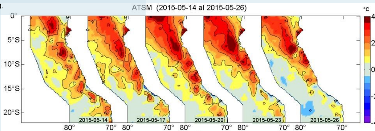
Figura 2. Anomalías de la temperatura superficial del agua ( ^{\circ}\text{C} ) en el mar peruano los días 14, 17, 20, 23 y 26 de mayo. Datos: AVHRR/NOAA. Procesamiento: IMARPE.
