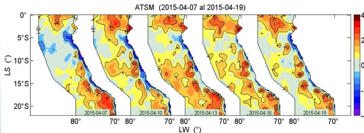
Figura 2. Anomalías promedio diarias de la temperatura superficial del agua (°C) en el mar peruano los días 07, 10, 13, 16 y 19 de abril (Fuente: Datos de AVHRR/NOAA; procesado por IMARPE).
