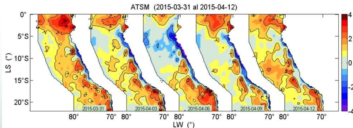
Figura 2. Anomalías promedio diarias de la temperatura superficial del agua (°C) en el mar peruano los días 31 de marzo, 03, 06, 09 y 12 de abril (Fuente: Datos de AVHRR/NOAA; procesado por IMARPE).
