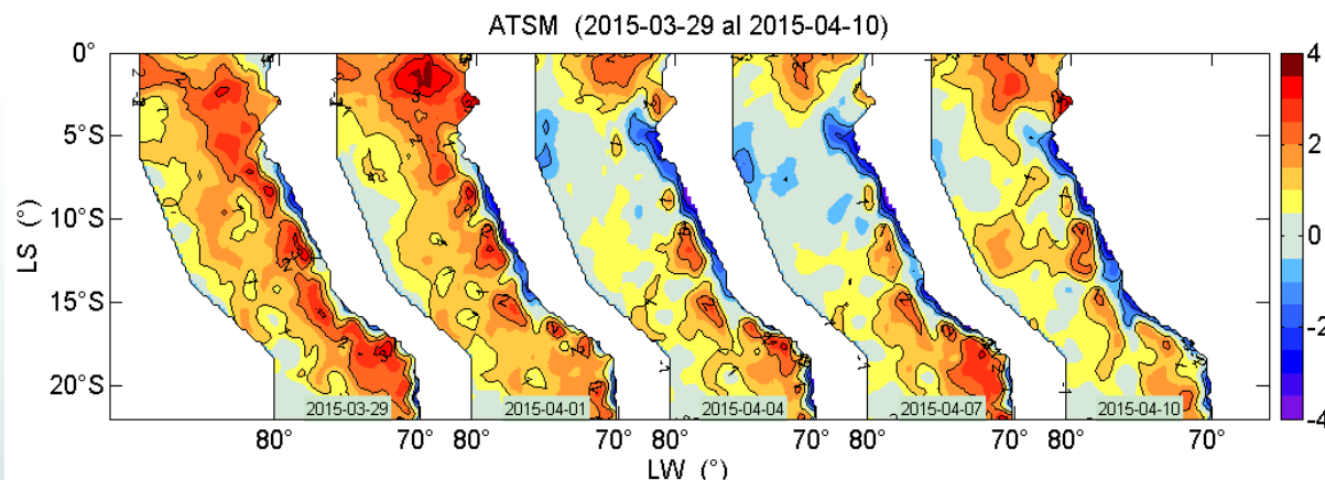
Figura 2. Anomalías promedio diarias de la temperatura superficial del agua (°C) en el mar peruano los días 29 de marzo y 01, 04, 07 y 10 de abril de 2015 (Fuente: Datos de AVHRR/NOAA. Procesamiento: IMARPE).
