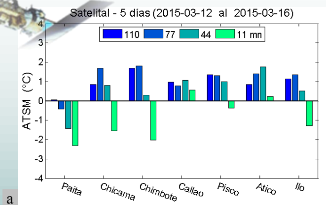
Figura 7. Promedios de las ATSM (°C), basados en: a) Observaciones satelitales en puntos de monitoreo ubicados a distancias aprox. de 110, 77, 44 y 11 millas náuticas (mn) de la costa y, b) Registros in situ del litoral costero.
