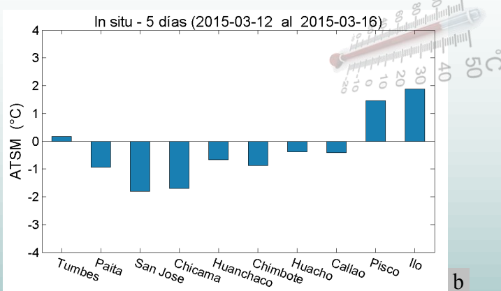
Figura 7. Promedios de las ATSM (°C), basados en: a) Observaciones satelitales en puntos de monitoreo ubicados a distancias aprox. de 110, 77, 44 y 11 millas náuticas (mn) de la costa y, b) Registros in situ del litoral costero.
