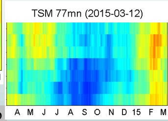
Figura 5. Diagramas Hovmöller de TSM (°C) durante un año, en puntos de monitoreo de información satelital a distancias de a) 110, b) 77, c) 44, d) 11 millas náuticas (mn) de la costa (puntos azules) y, e) en estaciones costeras registradas por IMARPE (puntos rojos).
