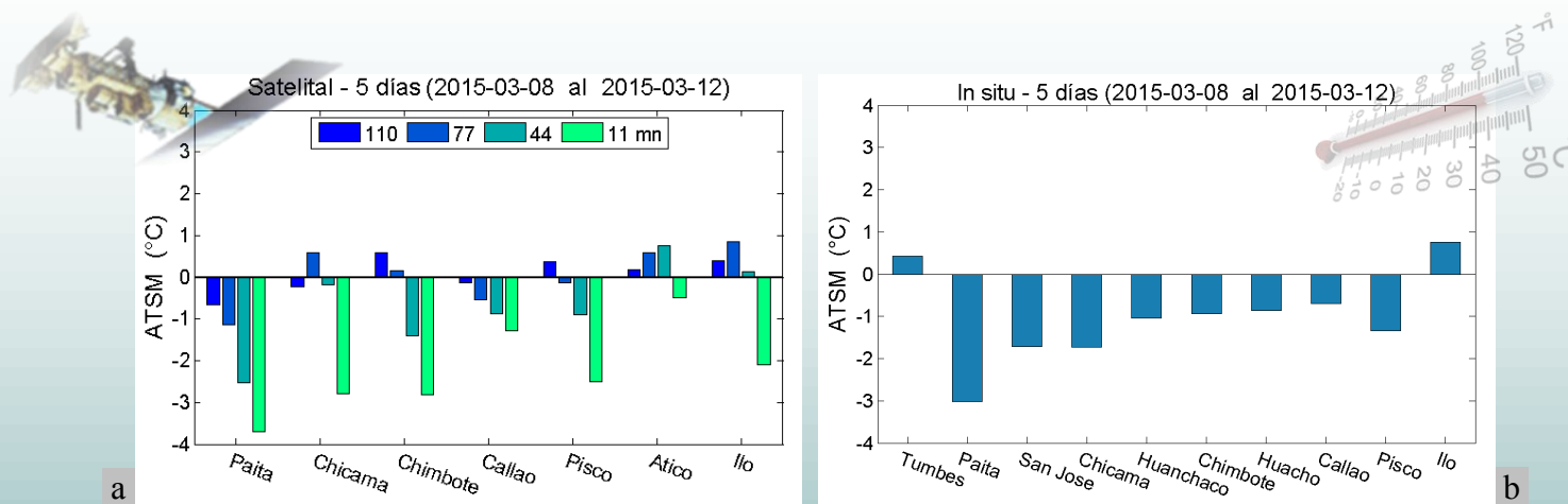
Figura 7. Promedios de las ATSM (°C), basados en: a) Observaciones satelitales en puntos de monitoreo ubicados a distancias aprox. de 110, 77, 44 y 11 millas náuticas (nm) de la costa y, b) Registros in situ del litoral costero.
