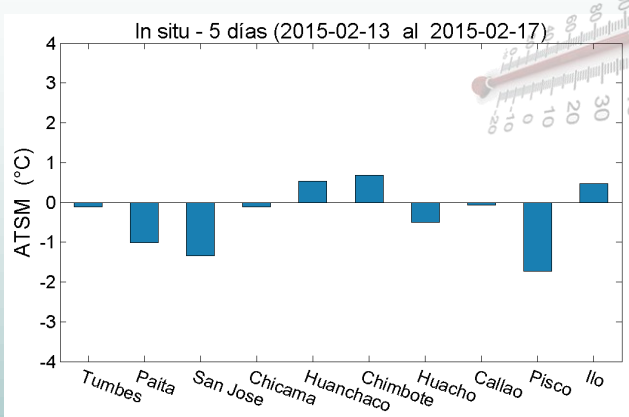
Figura 7. Promedios de las ATSM (°C), basados en: a) Observaciones satelitales en puntos de monitoreo ubicados a distancias aprox. de 110, 77, 44 y 11 millas náuticas (mn) de la costa y, b) Registros in situ del litoral costero.
