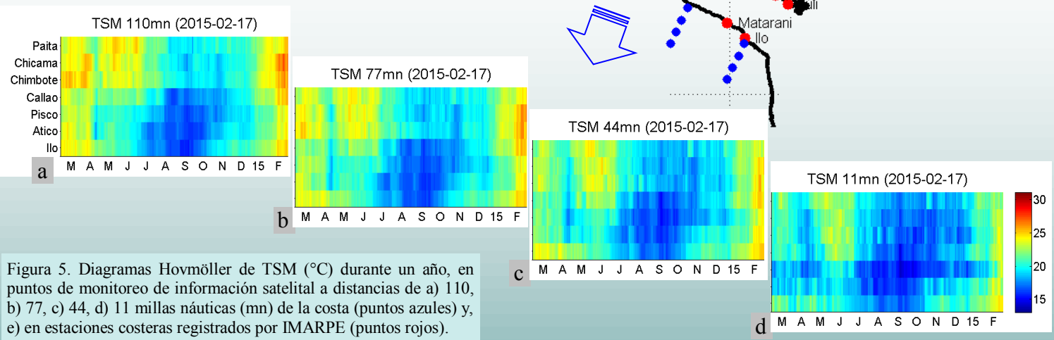
Figura 5. Diagramas Hovmöller de TSM (°C) durante un año, en puntos de monitoreo de información satelital a distancias de a) 110, b) 77, c) 44, d) 11 millas náuticas (mn) de la costa (puntos azules) y, e) en estaciones costeras registrados por IMARPE (puntos rojos).
