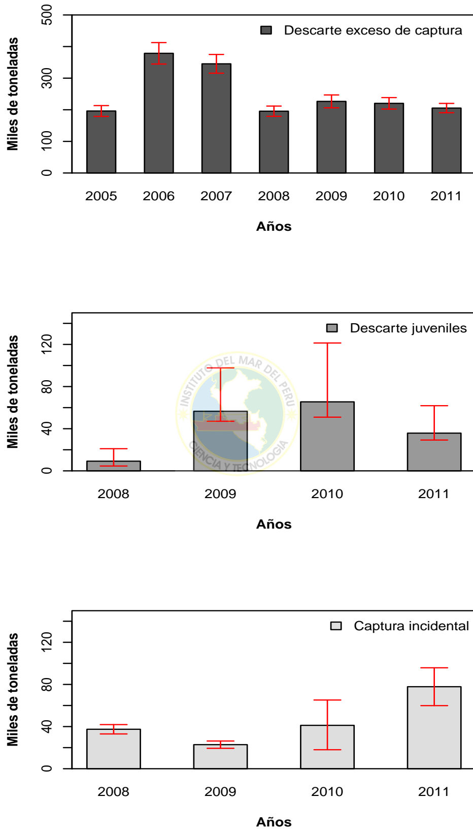
Figura 27. Estimación del descarte por exceso de captura, descarte de juveniles y captura incidental en la pesquería industrial de cerco del stock norte-centro de la anchoveta peruana obtenidos mediante el Modelo Delta.
