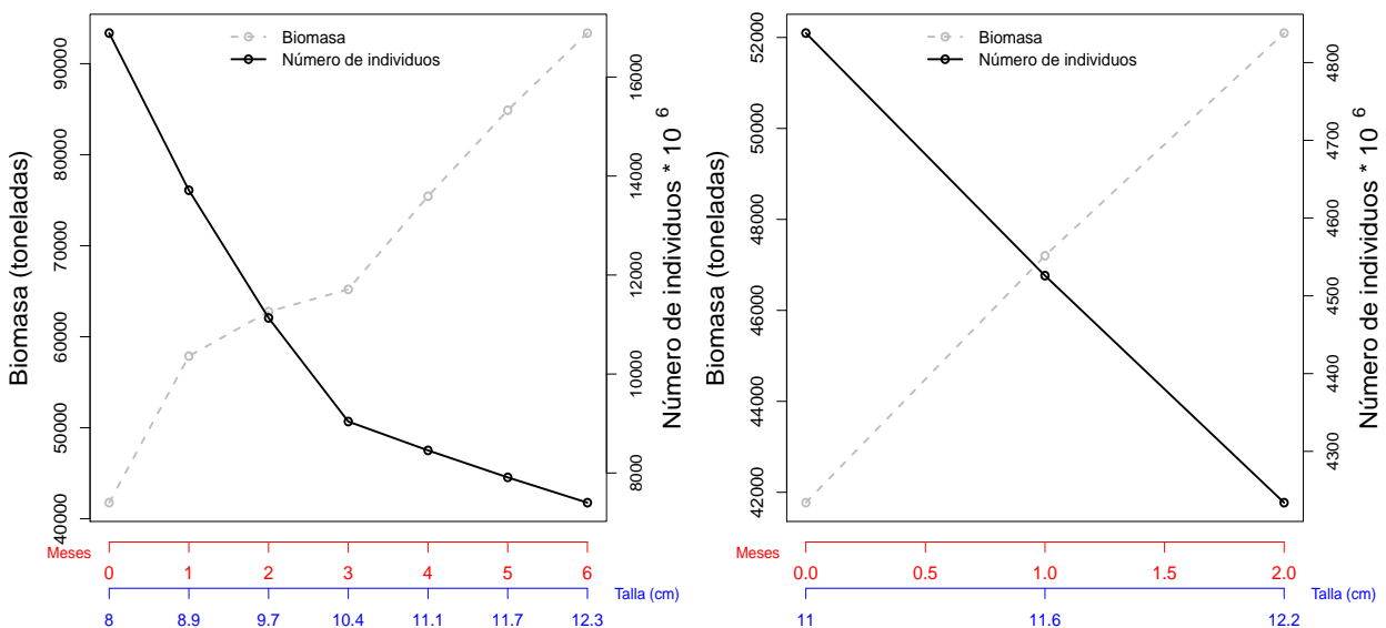
Figura 30. Proyección de biomasa y de número de individuos a partir de individuos de 8 cm de longitud (panel izquierdo) y de 11 cm. (panel derecho) hasta llegar a alcanzar la talla adulta (> 12 cm.)
