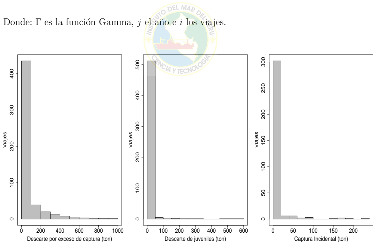
Figura 8. Histograma de frecuencia para el descarte por exceso de captura, descarte de juveniles y captura incidental en la pesquería industrial de cerco del stock norte-centro de la anchoveta peruana, durante el periodo 2005 - 2011.
