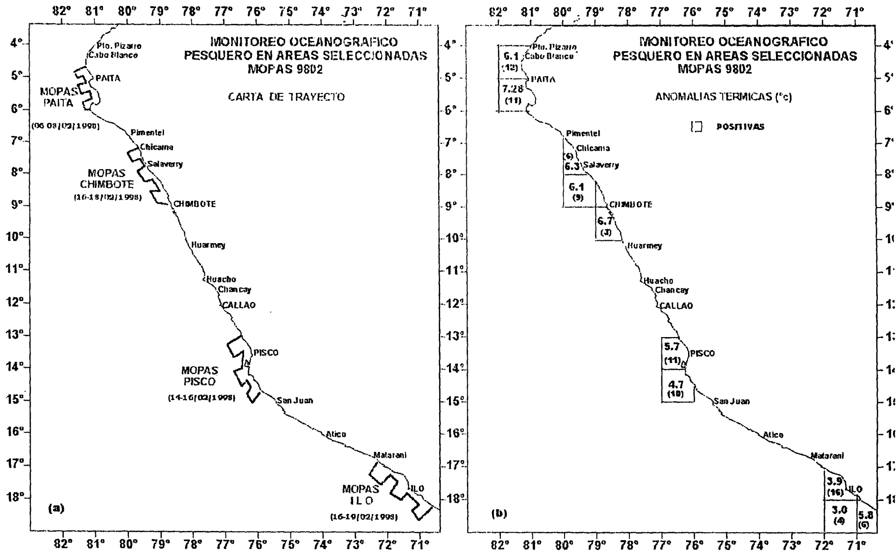
FIGURA 1. Cobertura de la operación MOPAS 9802 (a) y anomalías térmicas (°C) respecto al promedio patrón de febrero (b).
