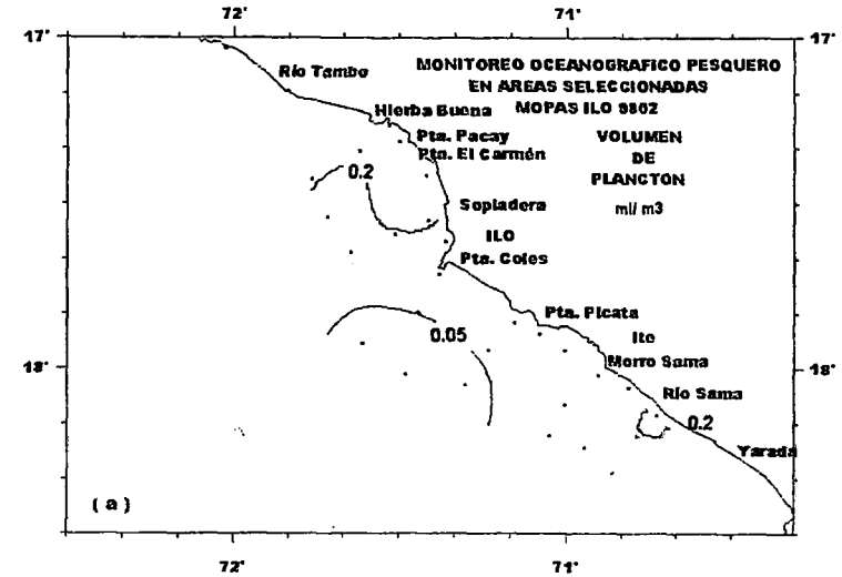
FIGURA 27. Volumen de plancton. MOPAS-Ilo.
