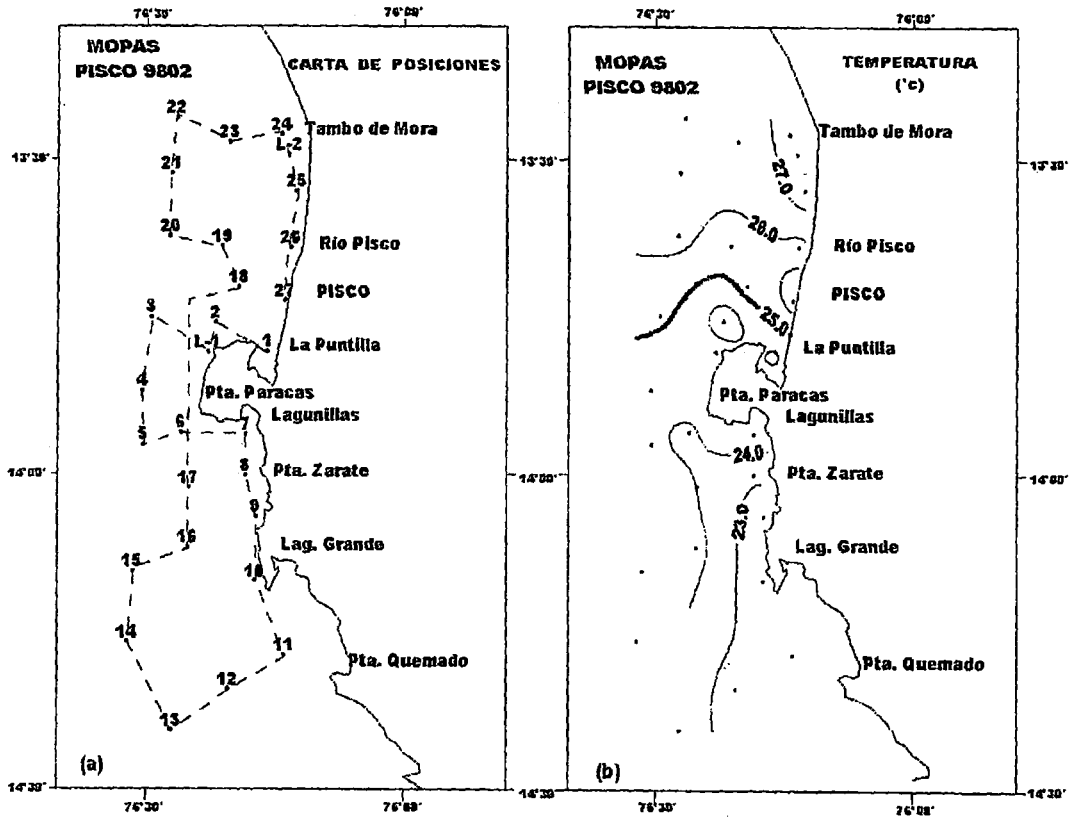
FIGURA 17. Carta de posiciones a) y distribución de la temperatura en la superficie del mar b). MOPAS-PISCO.
