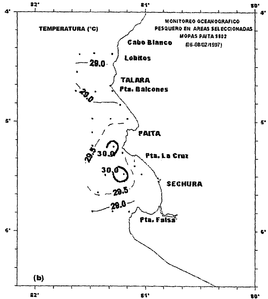
FIGURA 2. Carta de posiciones (a) y distribución de temperatura superficial del mar (b). MOPAS de Paita.
