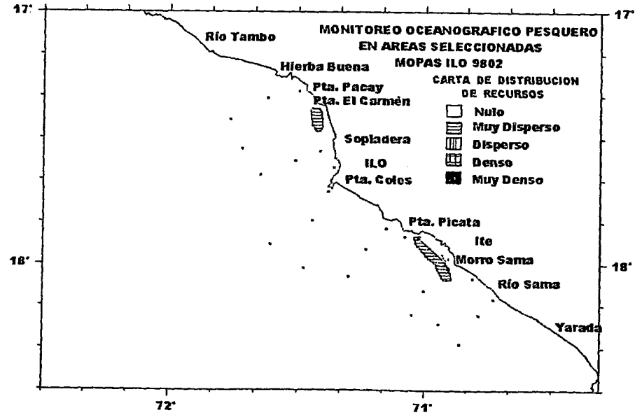
FIGURA 30. Distribución de recursos costeros. MOPAS-Ilo. E/P Iñeos Unidos.
