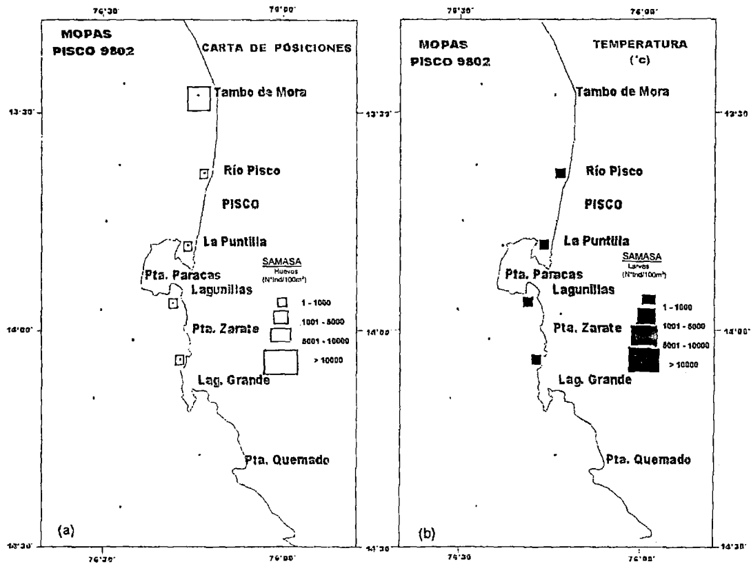
FIGURA 22. Distribución y abundancia de a) huevos y b) larvas de Engraulidae: Anchoa nasus "samasa". MOPAS-Pisco.
