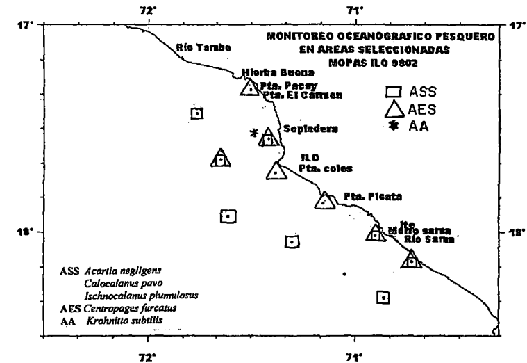
FIGURA 28. Distribución de indicadores de masa de agua del zooplancton. MOPAS-Ilo.
