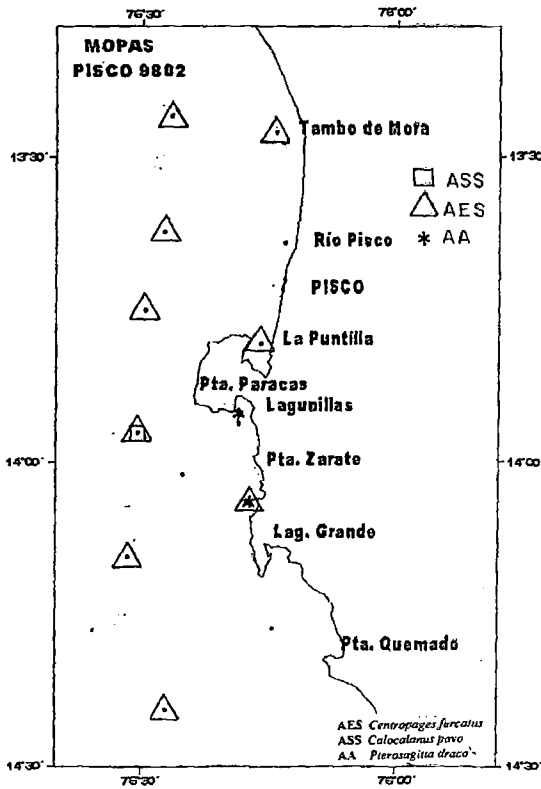
FIGURA 21. Distribución de indicadores de masas de agua del zooplancton. MOPAS-Pisco.
