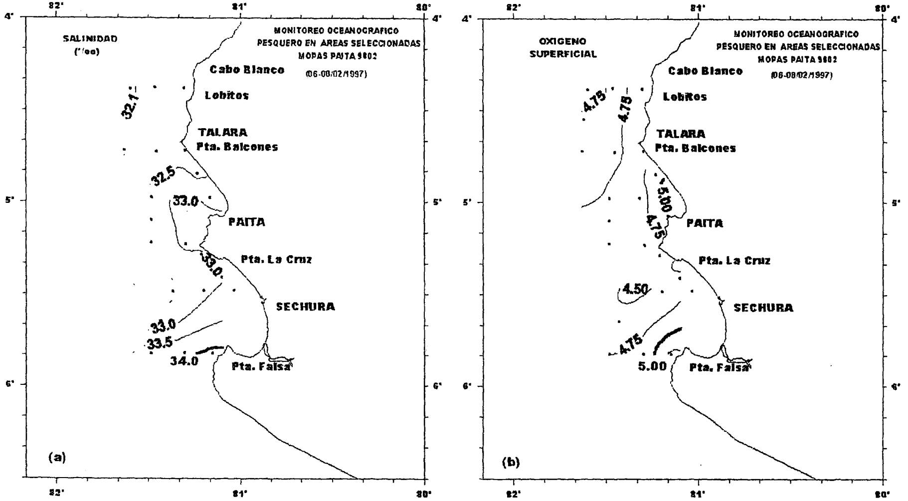
FIGURA 3. Distribución de la salinidad (a) y oxígeno (b) en la superficie del mar. MOPAS-Paita.
