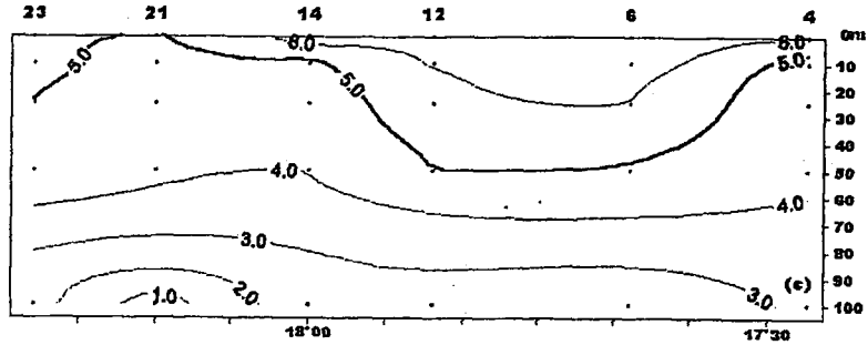
FIGURA 26. Secciones verticales de temperatura a), salinidad b) y oxígeno c) alrededor de las 15 mn frente a Ilo, con datos del MOPAS-Ilo.
