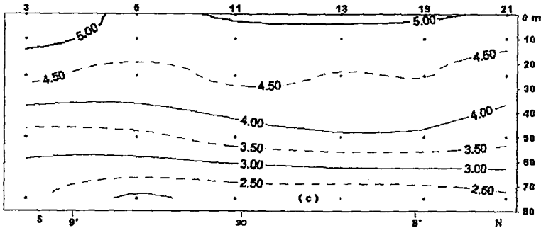
FIGURA 12. Secciones verticales de temperatura a) y salinidad b) y oxígeno c) alrededor de las 15 mn frente a Chimbote, con datos del MOPAS-Chimbote.
