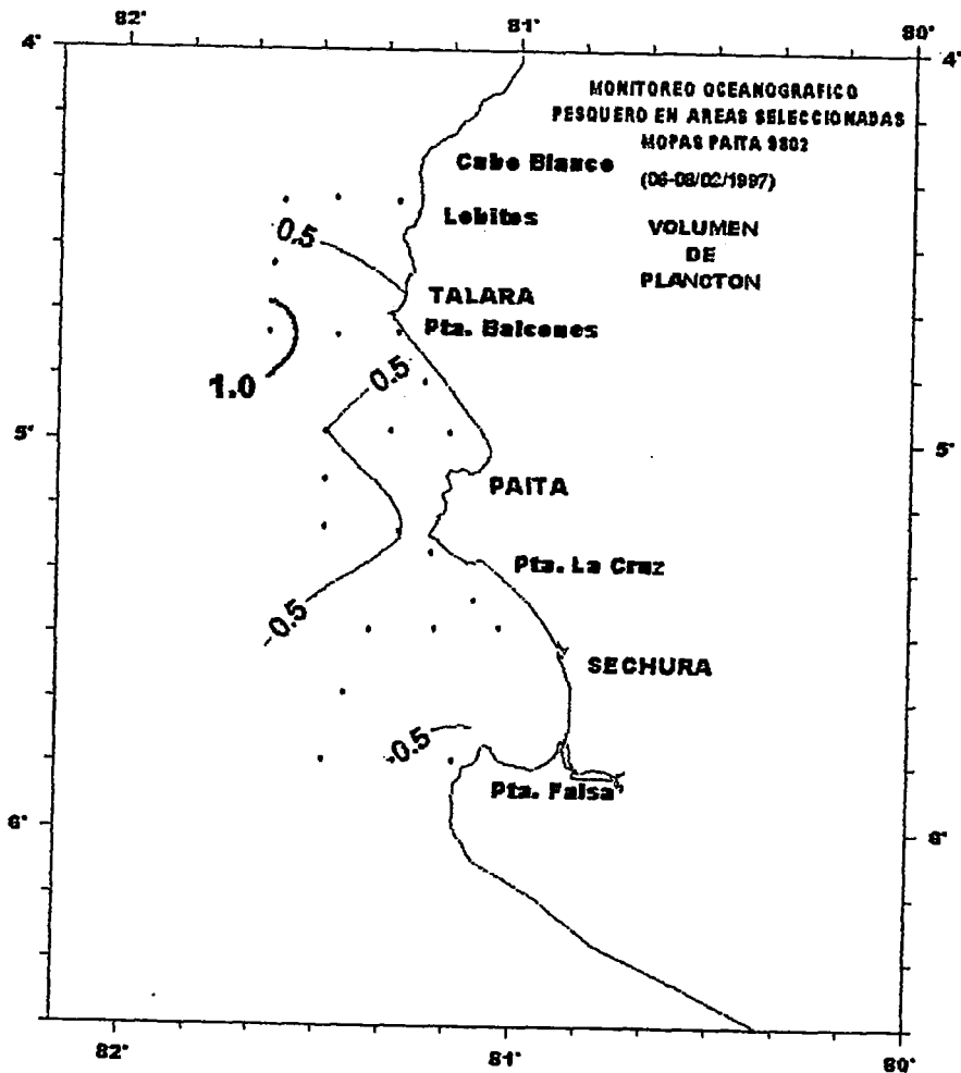
FIGURA 6. Volumen de plancton. MOPAS-Paita.
