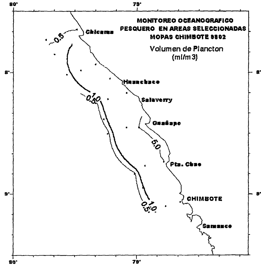
FIGURA 13. Volumen de plancton. MOPAS-Chimbote.
