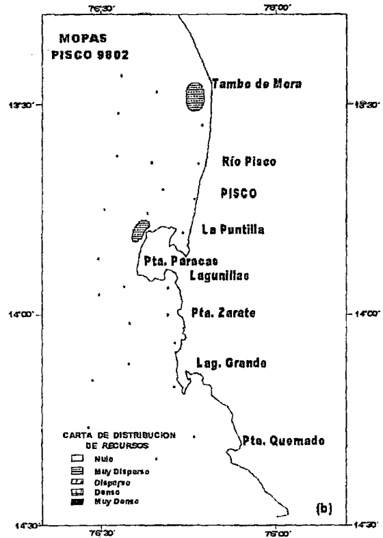
FIGURA 23. Distribución de recursos costeros. MOPAS-Pisco.
