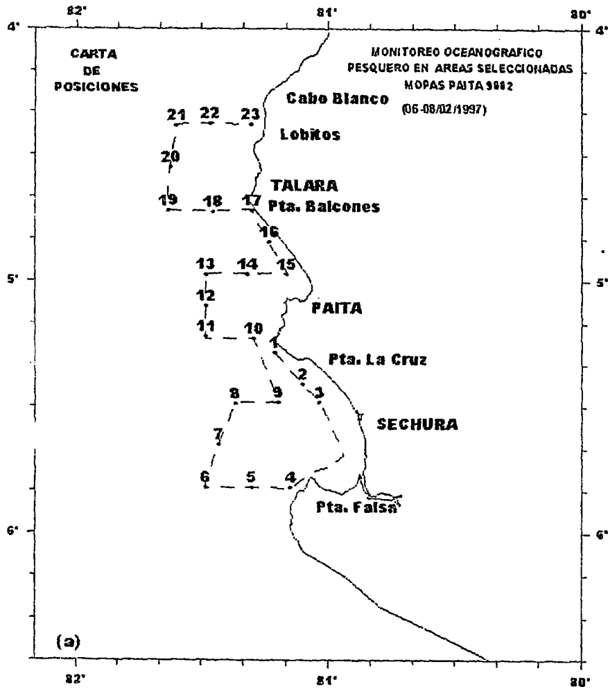
FIGURA 2. Carta de posiciones (a) y distribución de temperatura superficial del mar (b). MOPAS de Paita.
