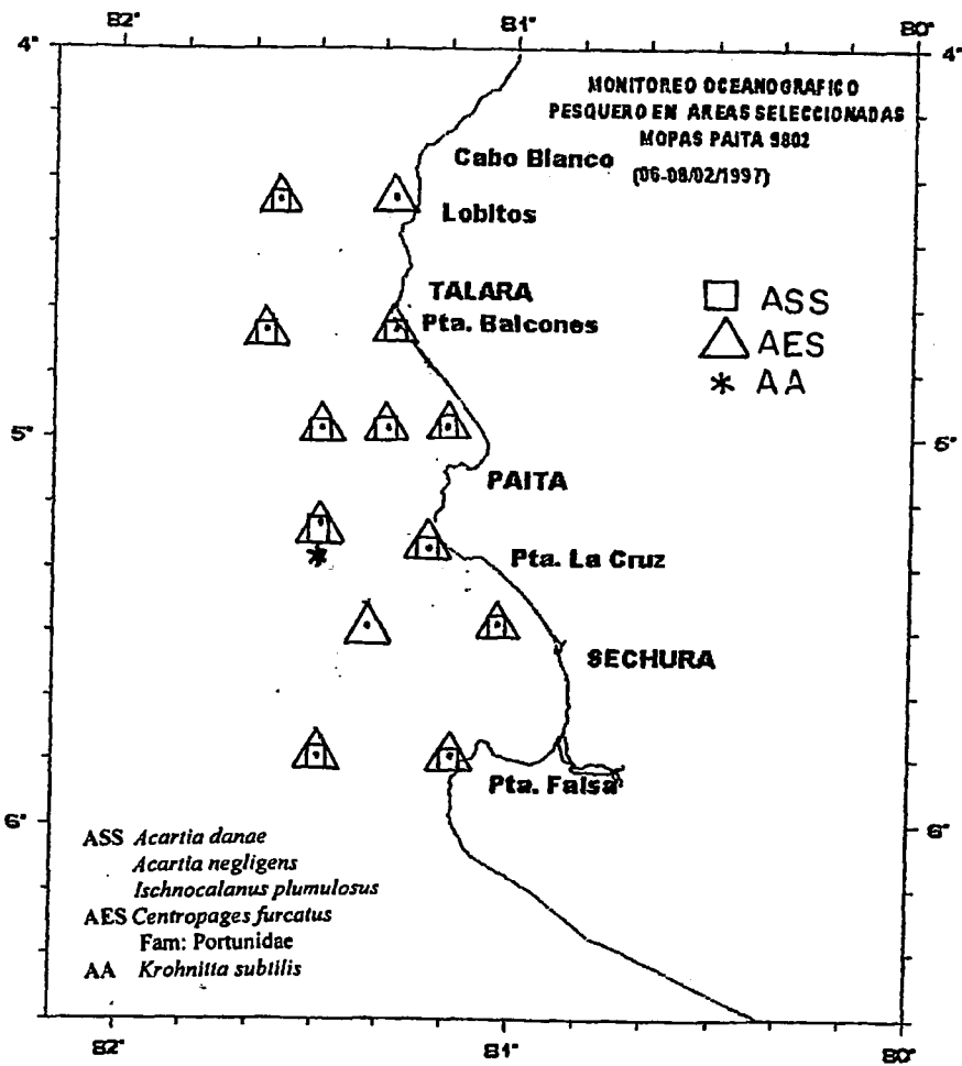
FIGURA 7. Distribución de indicadores de masas de agua del zooplancton MOPAS-Paita.
