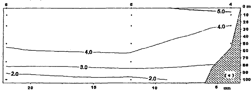
FIGURA 5. Perfil oceanográfico de temperatura (a), salinidad (b) y oxígeno c) frente a Punta Falsa, con datos del MOPAS-Paíta.
