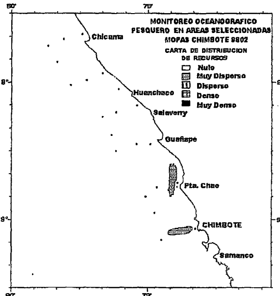
FIGURA 16. Distribución de zonas de pesca. MOPAS-Chimbote.
