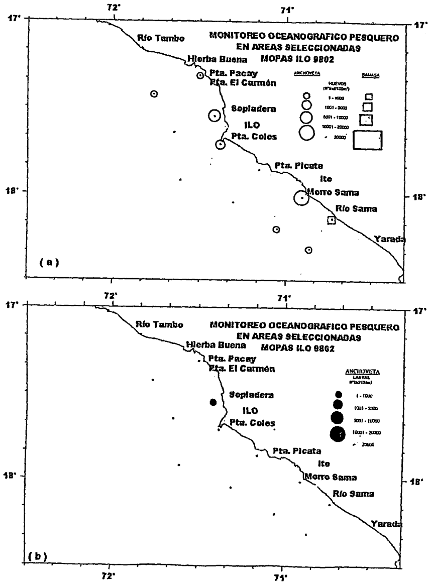
FIGURA 29. Distribución y abundancia de a) huevos y b) larvas de anchoveta. MOPAS-Ilo.
