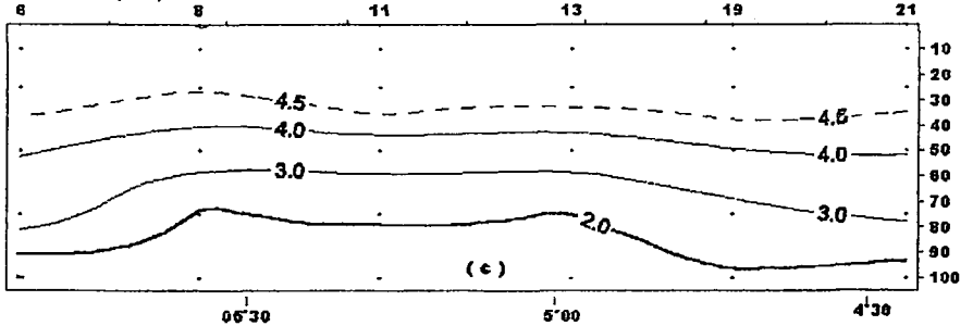
FIGURA 4. Secciones verticales de temperatura (a), salinidad (b) y oxígeno c), alrededor de las 15 mn frente a Paíta, con datos del MOPAS-Paíta.
